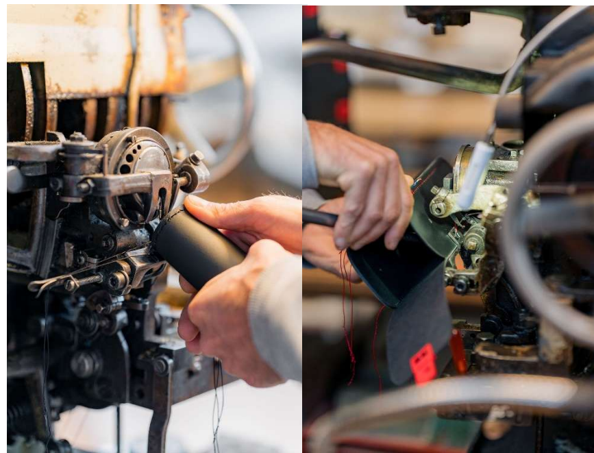
Le mécanisme alène + aiguille-crochet
